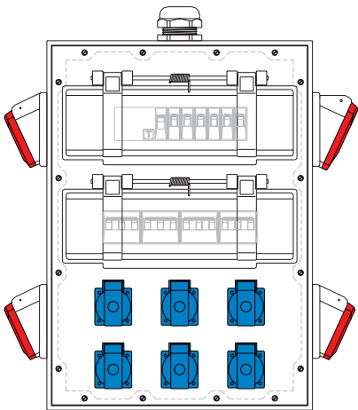
EDP-No.: 48422 Drawing-No.: 9714324
