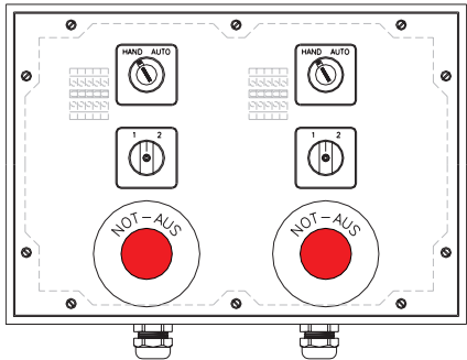
EDP-No.: 49138 Drawing-No.: 9714455
