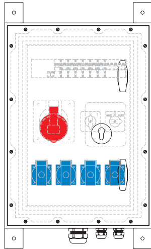
EDP-No.: 77491 Drawing-No.: 0520951
