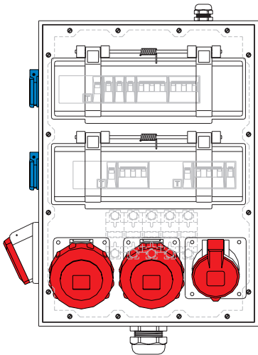
EDP-No.: 49139 Drawing-No.: 9714456
