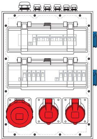
EDP-No.: 48144 Drawing-No.: 9714269
