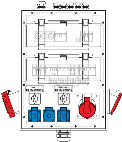
EDP-No.: 46169 Drawing-No.: 9613824
