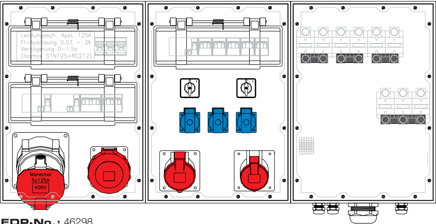
EDP-No.: 46298 Drawing-No.: 9613825
