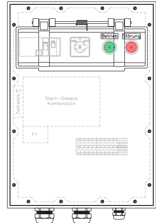
EDP-No.: 49147 Drawing-No.: 9714454
