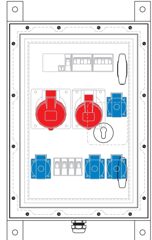
EDP-No.: 77492 Drawing-No.: 0520952
