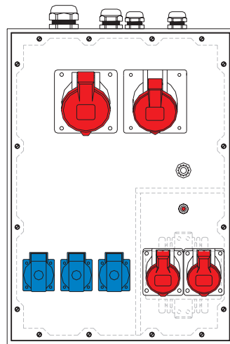
EDP-No.: 45816 Drawing-No.: 9613918
