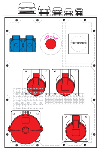
EDP-No.: 42315 Drawing-No.: 9513051
