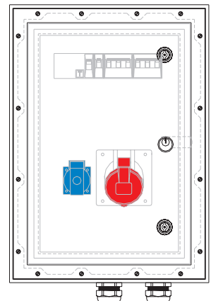
EDP-No.: 77493 Drawing-No.: 0520953
