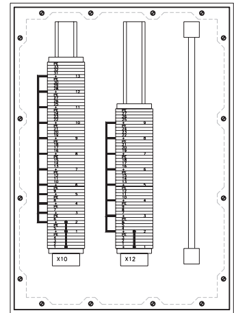
EDP-No.: 47319 Drawing-No.: 9714025
