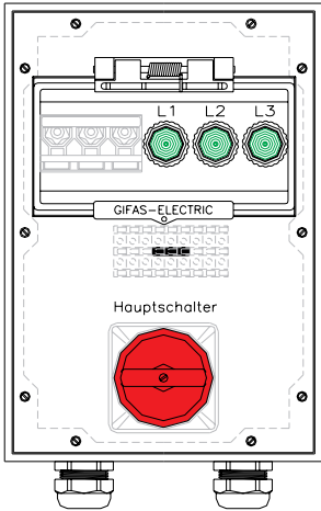
EDP-No.: 46320 Drawing-No.: 9613828
