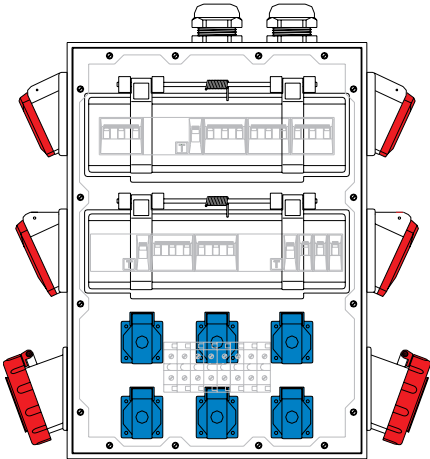
EDP-No.: 49146 Drawing-No.: 9714452
