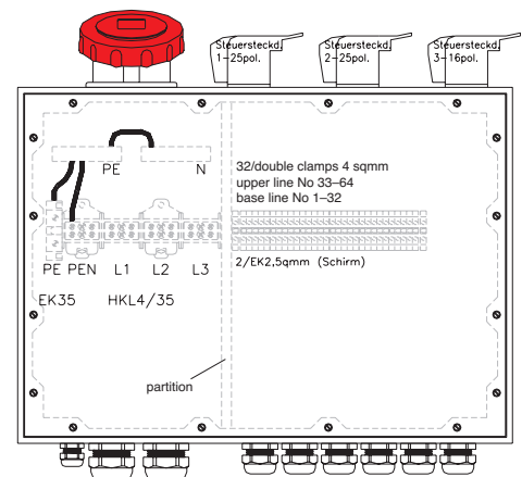
EDP-No.: 42560 Drawing-No.: 9513092
