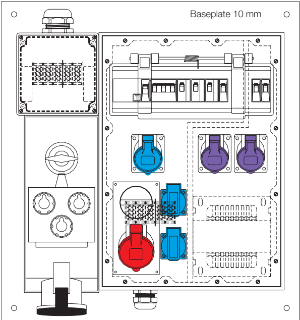
EDP-No.: 77332 Drawing-No.: 0520889
