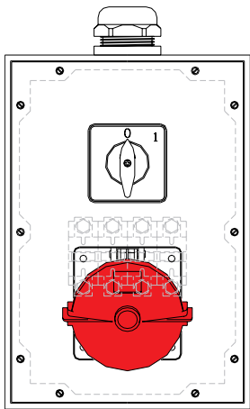
EDP-No.: 39502 Drawing-No.: 9513124
